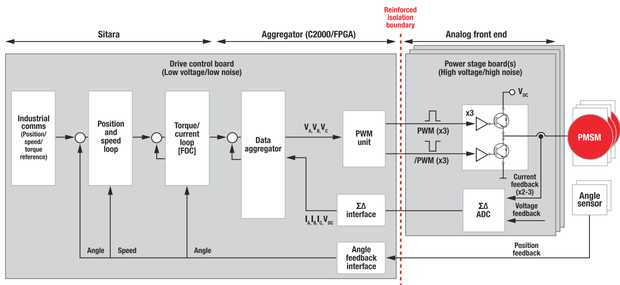
圖 3. 將 Sitara 處理器/微控制器做為伺服處理器，並將控制功能分擔給 C2000™ 微控制器或系統冷側 FPGA 的範例
