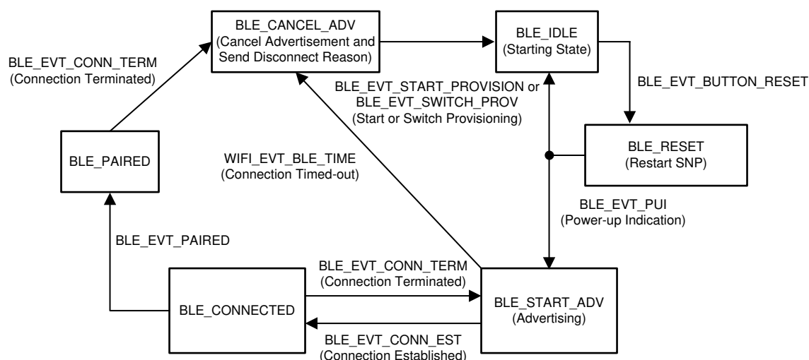
Figure 2-9. BLE Provisioning State Machine
