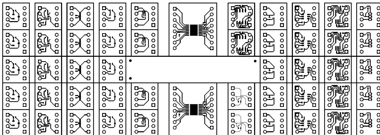
Figure 3-4. Top Layer
