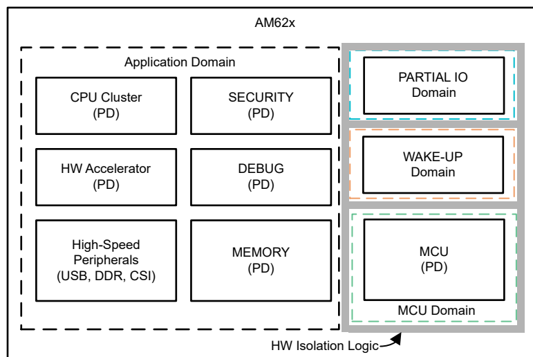
Abbildung 3-1. SoC-Partition
