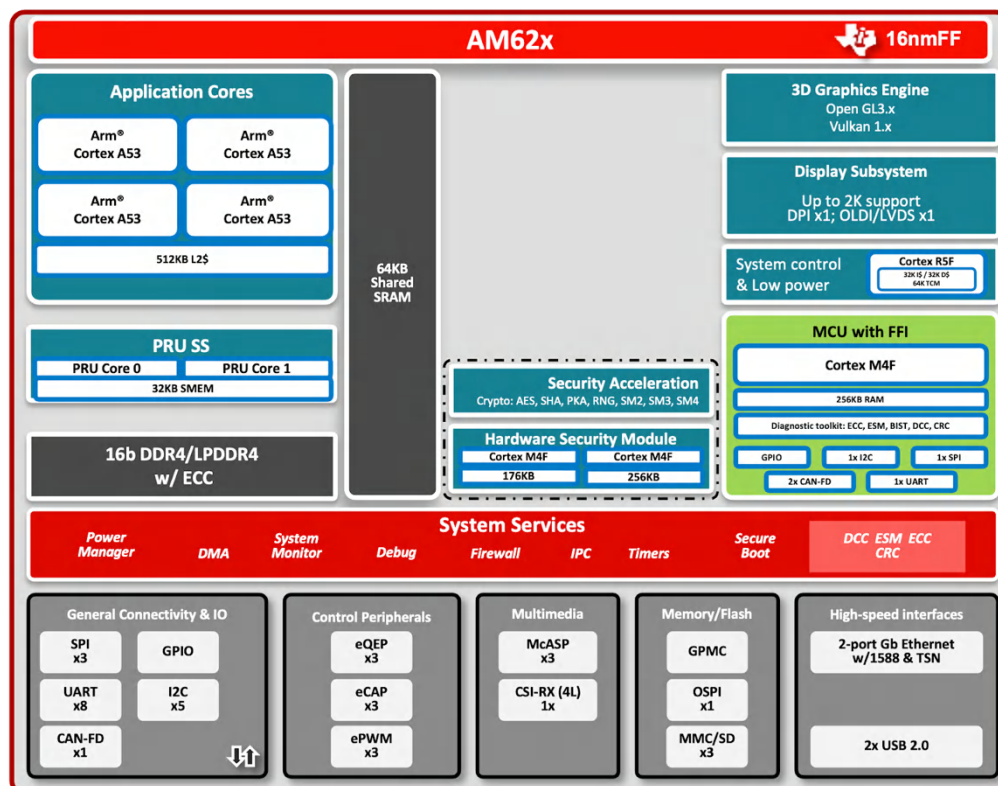
Abbildung 1-1. Blockschaftbild des AM62x-Prozessors Sitara™
