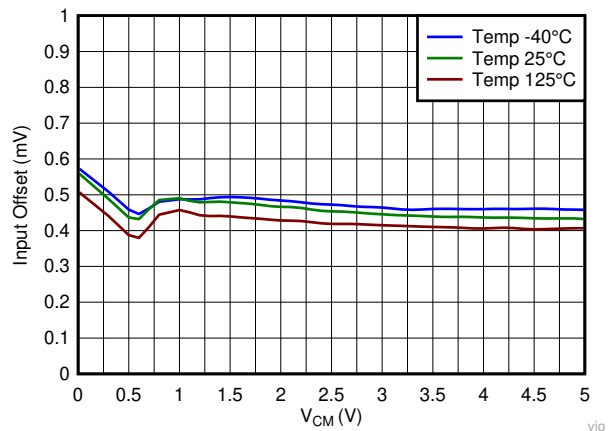
FIG 6-6. Input Offset Voltage vs V_{CM}
